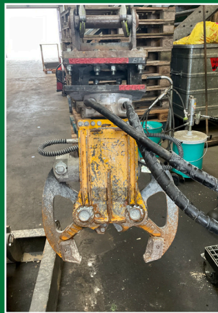
Abbruchzange / Pince de démolition
